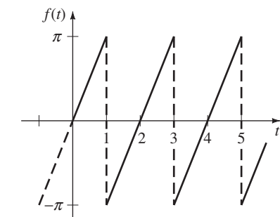
FIGURA 11.3.12 Función periódica forzada para el sistema resorte-masa.
