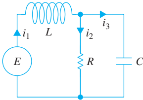
FIGURA 7.6.3 Red eléctrica.
