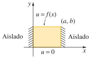
FIGURA 12.5.1 Temperaturas de estado estable en una placa rectangular.
