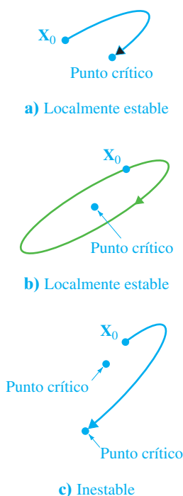
FIGURA 10.2.1 Puntos críticos.
