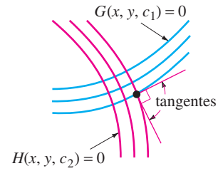
FIGURA 3.R.4 Trayectorias ortogonales.
