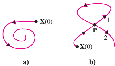
FIGURA 10.1.2 La curva en a) se llama arco.
