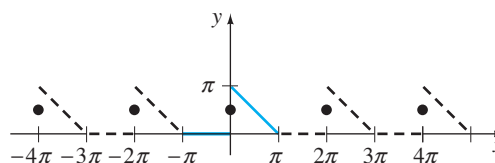
FIGURA 11.2.3 Extensión periódica de la función que se muestra en la figura 11.2.1. ■
