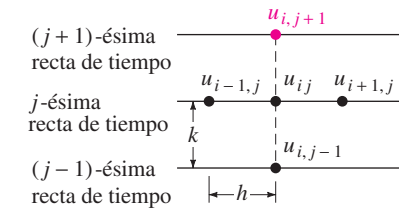
FIGURA 15.3.1 u en t = j + 1 se determina a partir de los tres valores de u en t = j y un valor en t = j - 1 .
