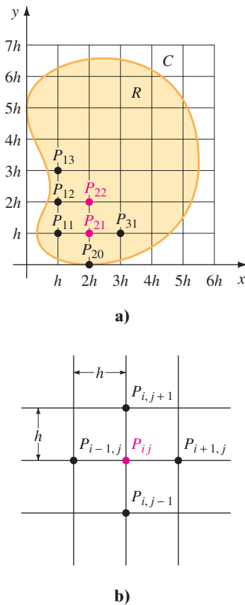
FIGURA 15.1.2 Malla rectangular sobrepuesta sobre la región R .
