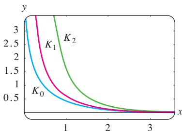
FIGURA 6.4.4 Funciones modificadas de Bessel de segunda clase para n = 0, 1, 2
