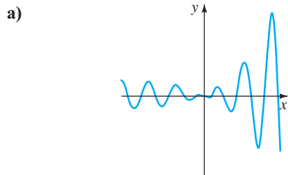
FIGURA 4.4.1 Curva solución.
