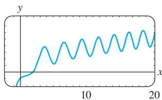
FIGURA 4.10.2 Curva solución numérica para el PVI en (1).
