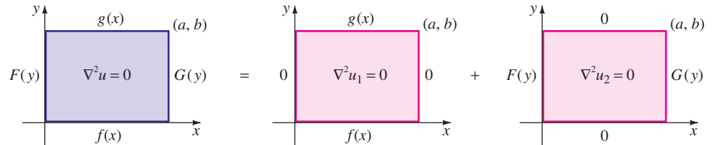
FIGURA 12.5.3 Solución u = \text{solución } u_1 \text{ del problema 1} + \text{solución } u_2 \text{ del problema 2.}
