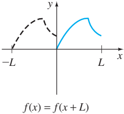
FIGURA 11.3.9 Reflexión identidad.
