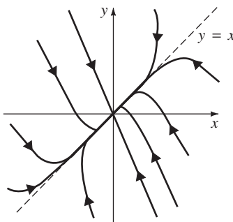
FIGURA 10.2.7 Nodo estable.
