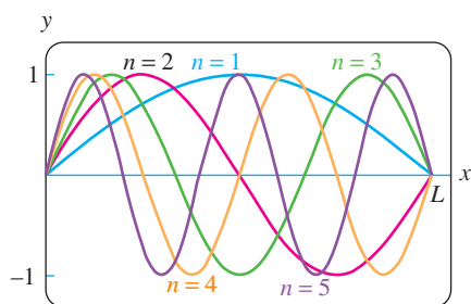
FIGURA 5.2.4 Gráficas de las eigenfunciones y_n = \sin(n\pi x/L) , para n = 1, 2, 3, 4, 5
