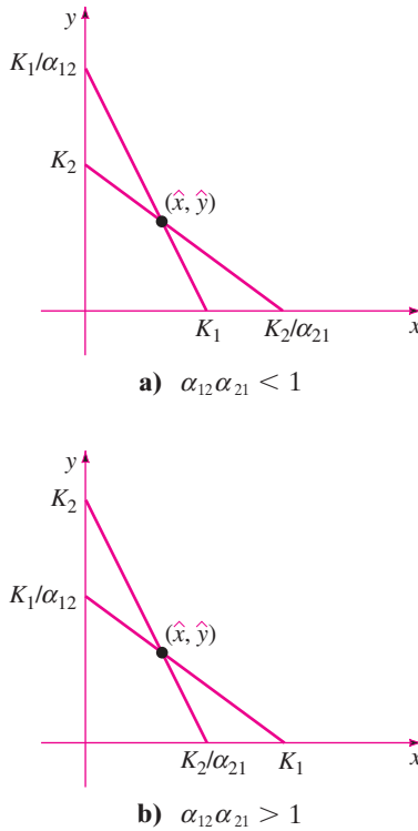
FIGURA 10.4.11 Dos condiciones cuando el punto crítico (\hat{x}, \hat{y}) está en el primer cuadrante.
