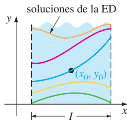
FIGURA 1.2.1 Solución del PVI de primer orden.
