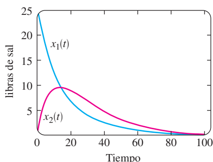
FIGURA 4.9.1 Libras de sal en los tanques A y B del ejemplo 3.
