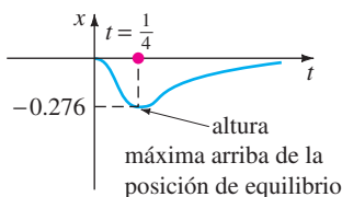
FIGURA 5.1.10 Sistema críticamente amortiguado del ejemplo 4.
