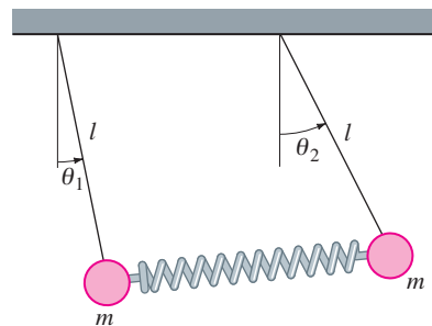
FIGURA 7.R.12 Péndulos acoplados del problema 47.
