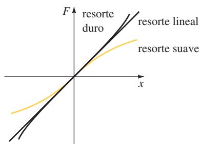
FIGURA 5.3.1 Resortes duros y suaves.
