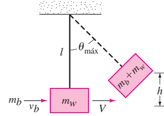
FIGURA 5.3.10 Péndulo balístico del problema 19.
