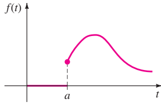
b) f(t-a)u(t-a)
