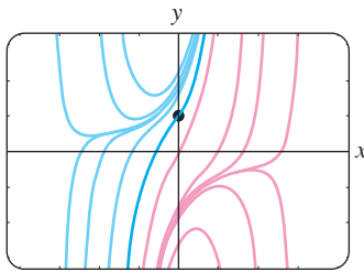
FIGURA 2.3.5 Curvas solución de la ED del ejemplo 7
