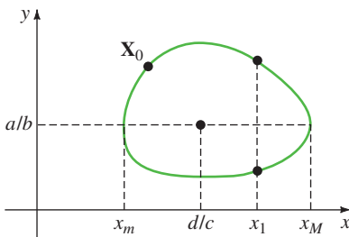
FIGURA 10.4.9 Solución periódica del modelo de Lotka-Volterra.
