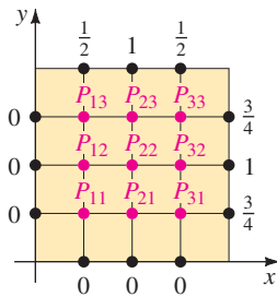
FIGURA 15.1.4 Región R del ejemplo 1 con más puntos de malla.
