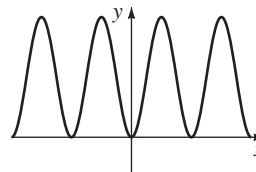
FIGURA 4.4.4 Curva solución.
