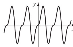
FIGURA 4.4.3 Curva solución.
