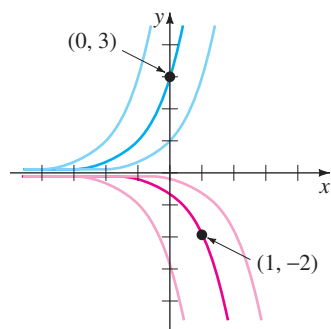
FIGURA 1.2.3 Soluciones de los dos PVI.
