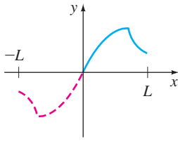
FIGURA 11.3.8 Reflexión impar.
