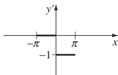
FIGURA 11.2.2 Derivada f' continua en partes del ejemplo 2.
