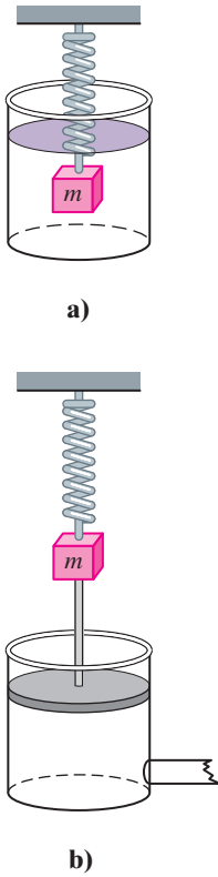
FIGURA 5.1.5 Dispositivos de amortiguamiento.
