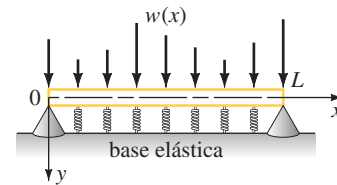
FIGURA 7.R.11 Viga sobre la base elástica del problema 46.
